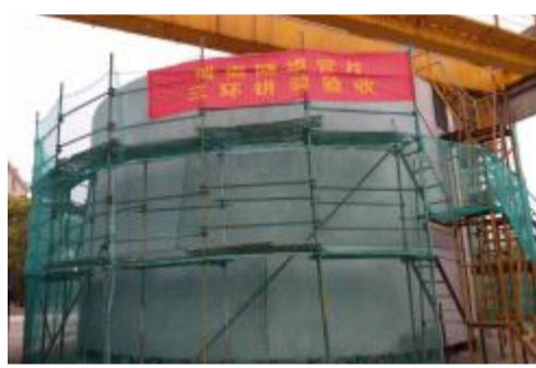
2018年4月4日上午，杭构·建工建材公司传来喜讯，自1月份开始试产的博奥过江隧道
